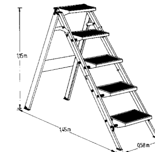
Little Jumbo 5 treden Werkhoogte 3.20 m Gewicht 12 kg Ingeklapt 174 x 55 x 7 cm
