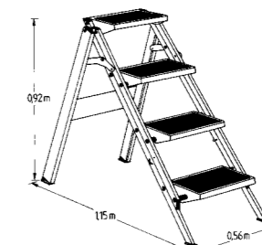
Little Jumbo 4 treden Werkhoogte 2.95 m Gewicht 10 kg Ingeklapt 145 x 55 x 7 cm
